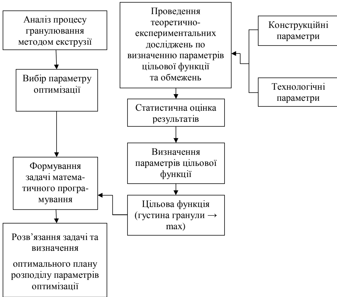
Рис. – Схема визначення оптимальних конструктивно-технологічних параметрів процесу грануляції дисперсних матеріалів ущільненням
