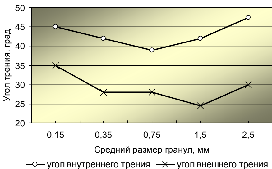
Рис. 4. Зависимость угла внутреннего и внешнего трения от среднего размера гранул
