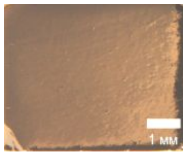
Рис. 5. Фотография кристалла CdZnTe, травленного в I 2 – ДМФА
