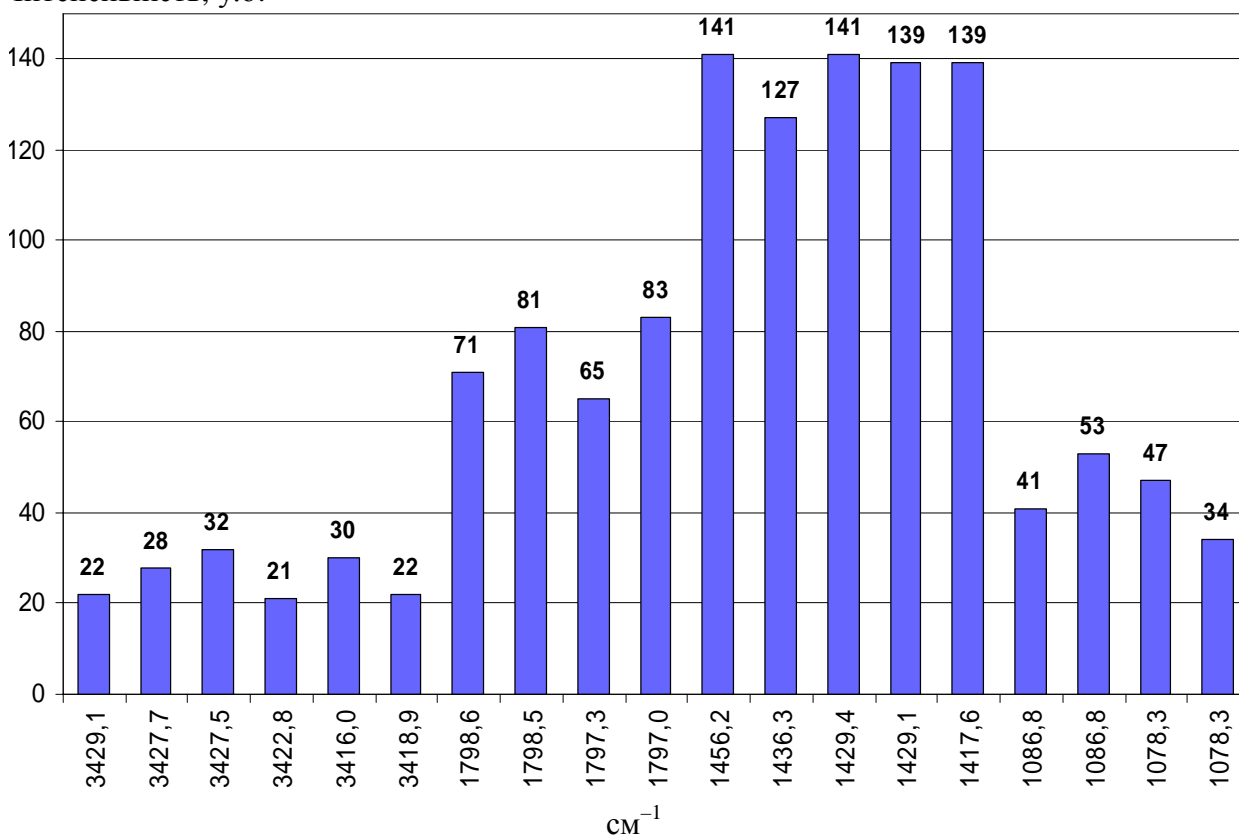
Рис. 2. Положення (см -1 ) та інтенсивність (у.о.) характеристичних смуг в ІЧ-спектрах вітчизняних і закордонних карбонатних наповнювачів:
