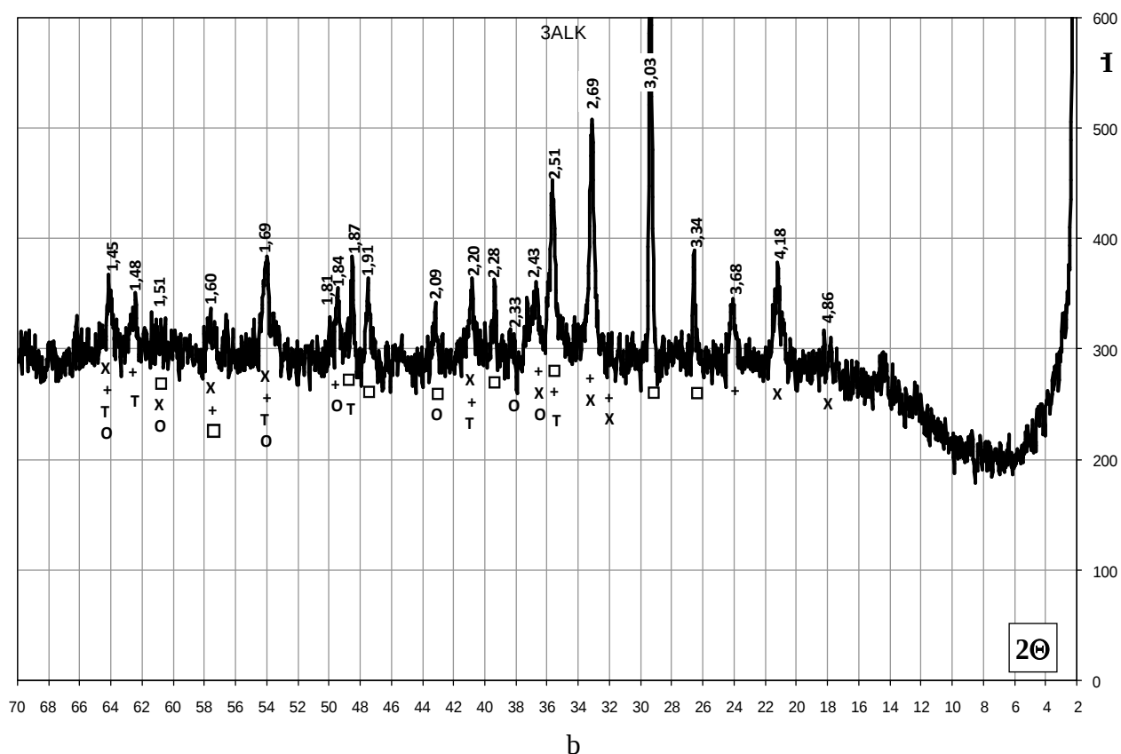
Рис. 1. Дифрактограми проб червоного шламу: а – МГЗ, б – ЗАЛК (х – гетит, + – гематит, т – рутил, о – гідраргиліт).
