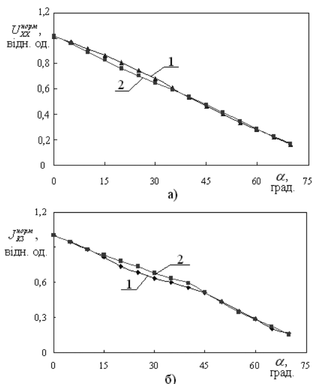
Рис. 2. Залежності U_{XX}^{norm}(\alpha) (а) та J_{KZ}^{norm}(\alpha) (б) у випадках опромінення БП Si-ФЕП нової генерації з боку p^+ - p переходу (1) та з боку випрямляючого переходу (2)
