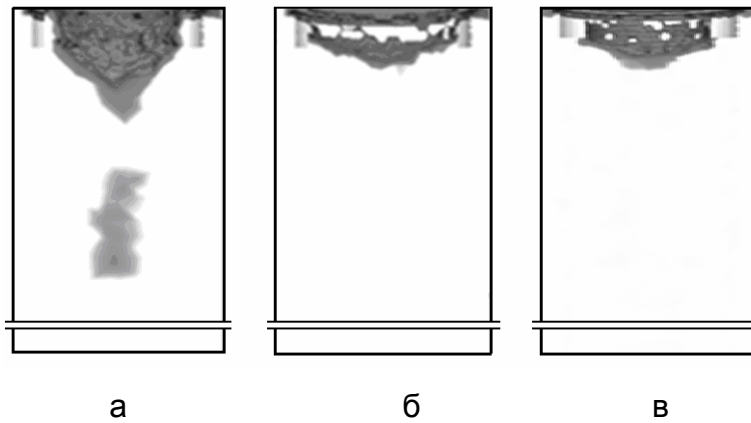
Рис.1. Схема распределения усадочных дефектов в слитке с прибыльной вставкой по существующей технологии (а), с ППВ при X=25 мм (б) и X=50 мм (в)
