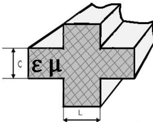
Рис.1. Оригинальная крестообразная линия передачи КВЧ диапазона.
